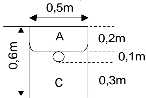
Tranchée d'épandage standard
